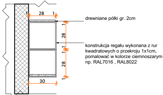
PRZEKRÓJ C-C
