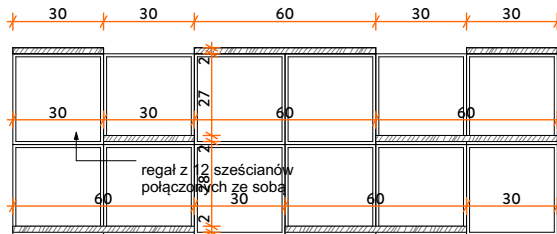
PRZEKRÓJ B-B
