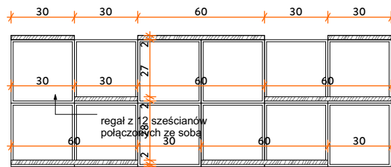
PRZEKRÓJ B-B
