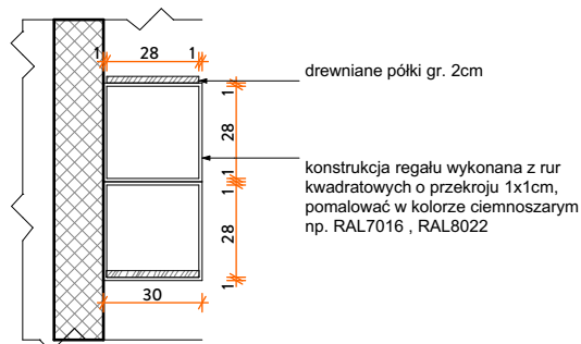
PRZEKRÓJ C-C
